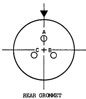
REAR GROMMET
