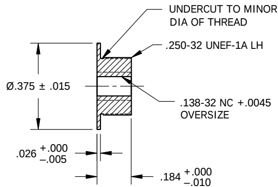
"-3", "-6" FLANGE
