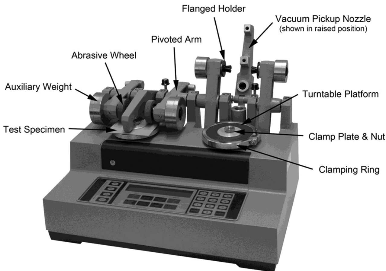
FIG. 1 Taber-Type Abraser
