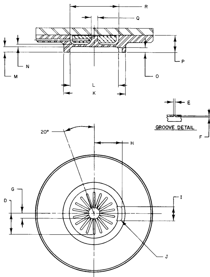
FIG. 4 Upper Die
