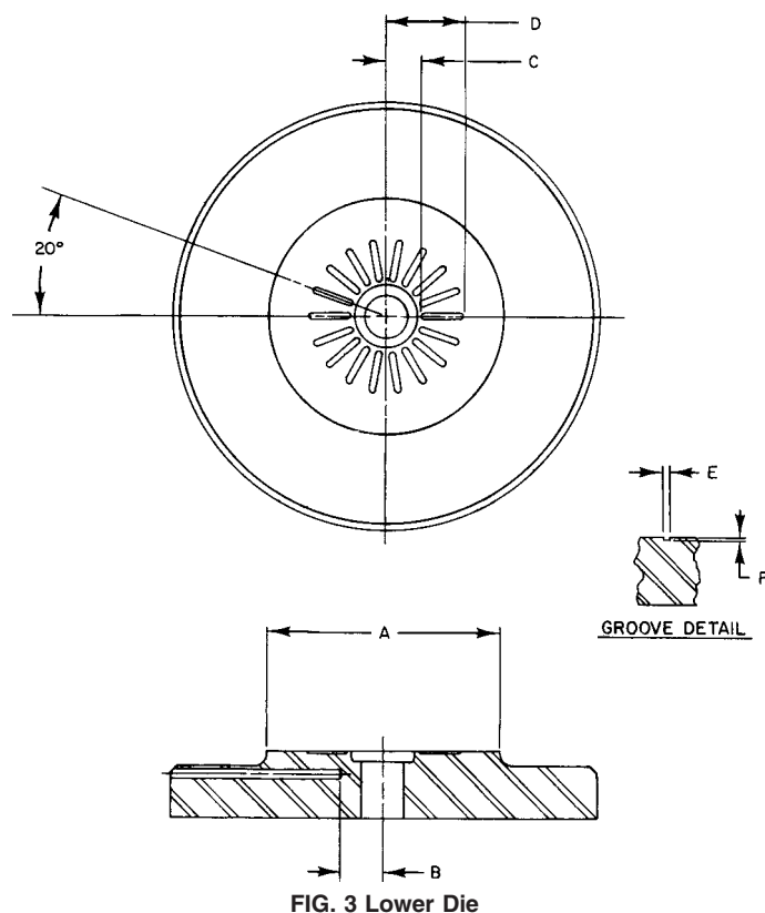
FIG. 3 Lower Die
