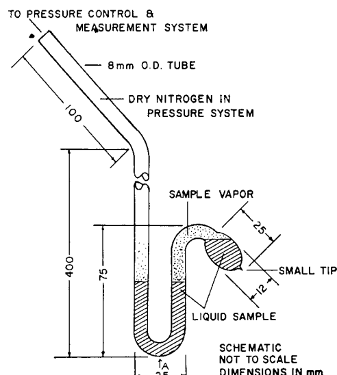
FIG. 1 Isoteniscope
