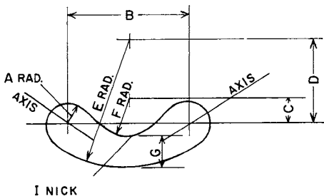
DIE A
