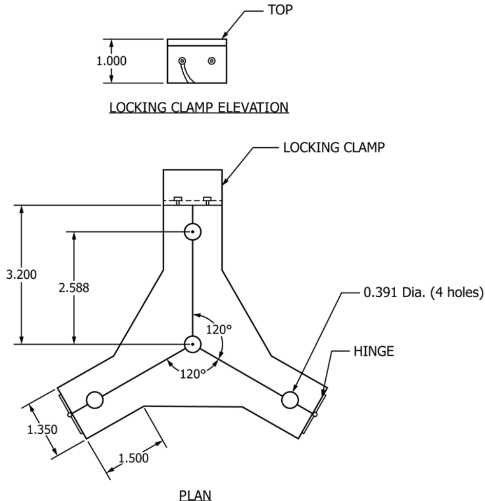
FIG. 2 MRP Guide Template
