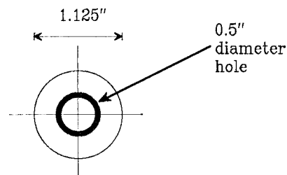
FIG. 1(d) Gasket Detail
