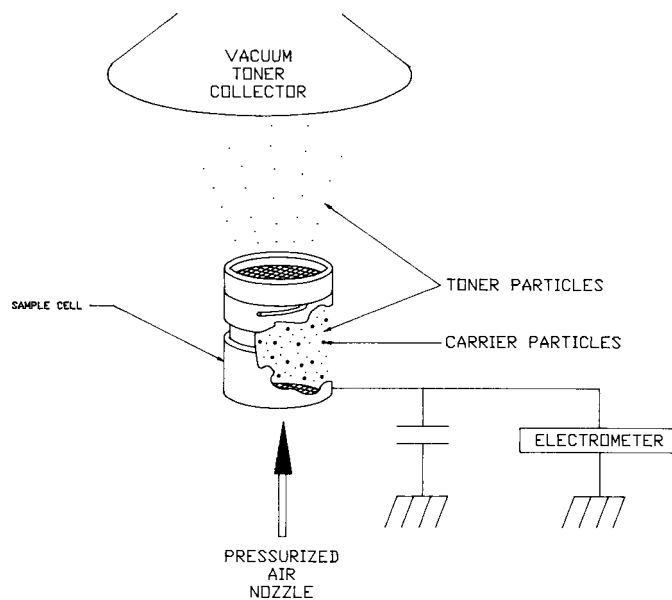
FIG. 2 Tribometer
