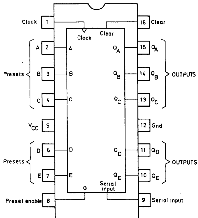
5-bit shift register
