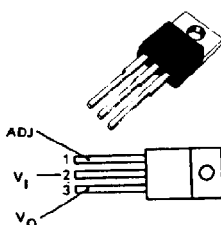
Boîtier F 138 (SP)
