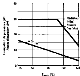
Courbe de décroissance Derating curve
