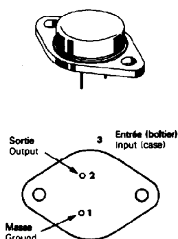
Boîtier F 24 (KM)
