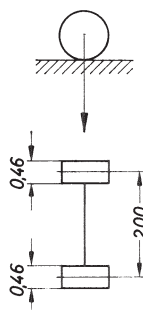
Bild 1. Maße der Regelfahrzeuge, Achsabmessungen und Radaufstandsbreiten in m
