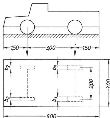
c) Lastkraftwagen (LKW)
