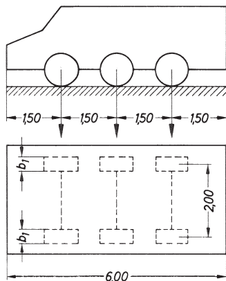
Bild 1. Maße der Regelfahrzeuge, Achsabmessungen und Radaufstandsbreiten in m
