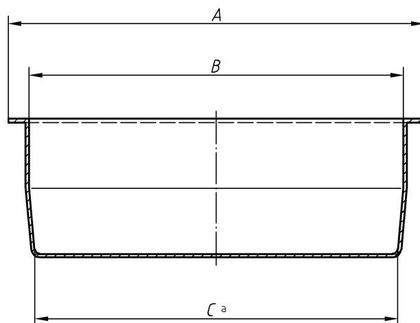
Bild 1 — Modul „60x40“
