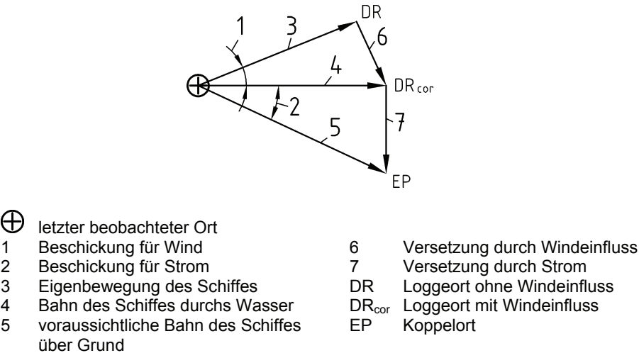
Bild 1 — Wind- und Stromversetzung
