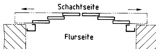
Bild 6: Horizontal bewegte, mittig öffnende, sechsblättrige (Teleskop-) Schacht-Schiebetür DIN 18 091 – 6 – H – M – T
