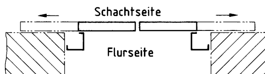
Bild 2: Horizontal bewegte, mittig öffnende, zweiblättrige Schacht-Schiebetür DIN 18 091 – 2 – H – M
