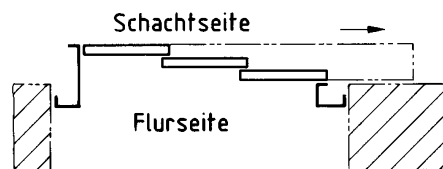
Bild 4: Horizontal bewegte, einseitig rechts öffnende, dreiblättrige (Teleskop-) Schacht-Schiebetür DIN 18 091 – 3 – H – R – T (einseitig links öffnende (Teleskop-) Schacht-Schiebetür spiegelbildlich)
