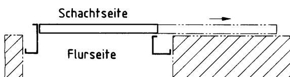
Bild 1: Horizontal bewegte, rechts öffnende, einblättrige Schacht-Schiebetür DIN 18 091 – 1 – H – R (links öffnende Schacht-Schiebetür spiegelbildlich)
