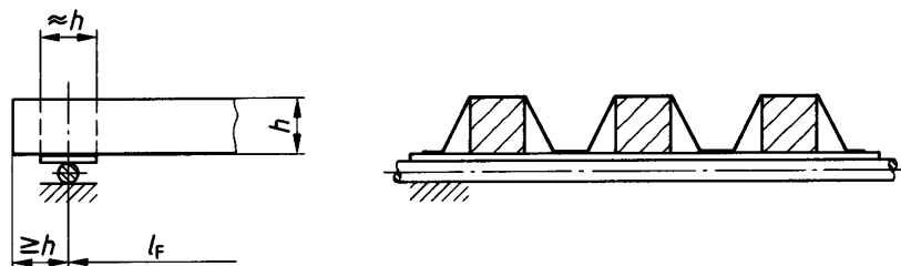
Bild 3. Auflagerausbildung beim Versuch „Feld“
