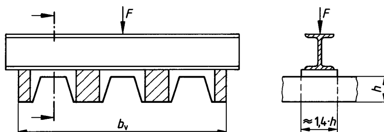
Bild 4. Beispiel für Lasteinleitung beim Versuch „Feld“
