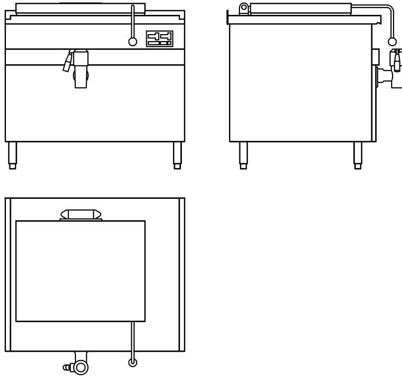
Bild 1 — Standbratpfanne
