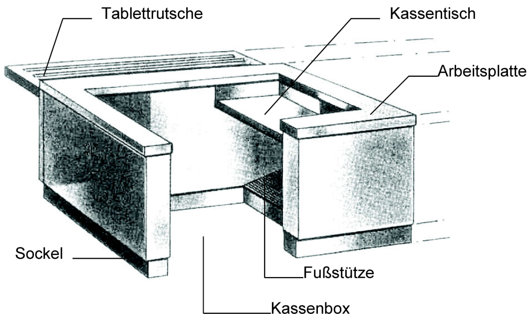
Bild 1 — Beispiel für ein Kassenmodul (in U-Form) (Warenzuführung links)
