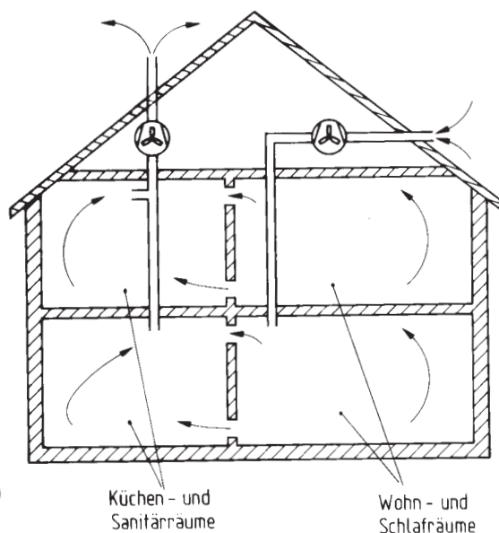
Bild 3: Maschinelle Lüftung — Be- und Entlüftungsanlage ohne Wärmerückgewinnung
