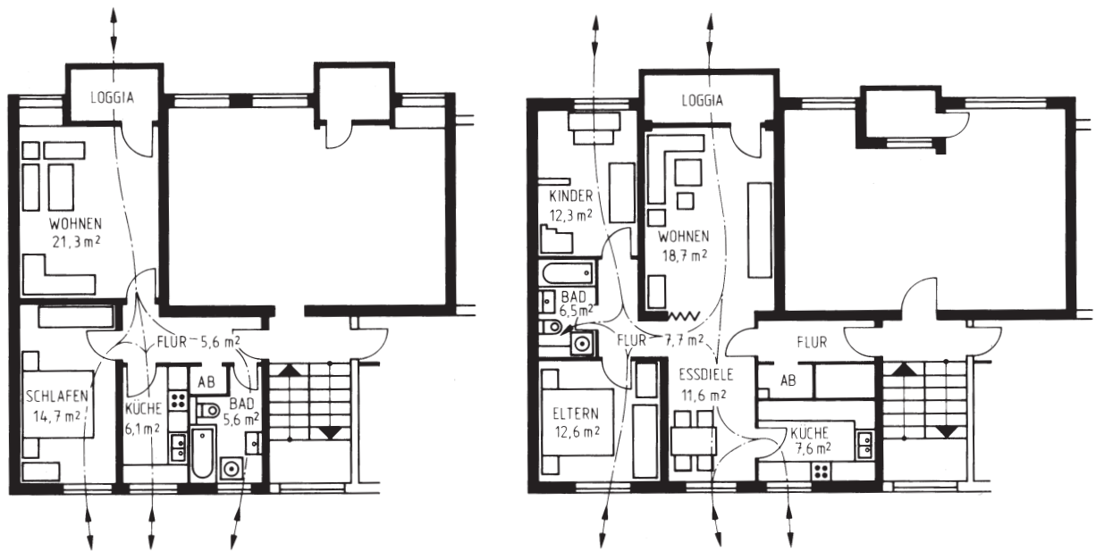
a) Querlüftung (Außenbad)
