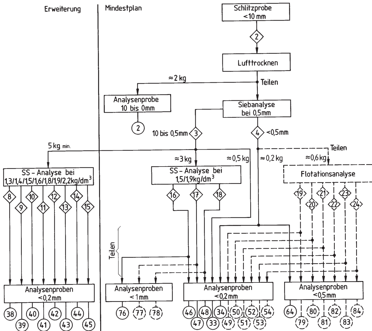
Bild 1. Schema der Vorbereitung und Untersuchung der Proben nach dem Mindestplan und dem erweiterten Plan
