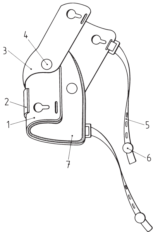
Bild 1: Knieschützer, Zusammenstellung
