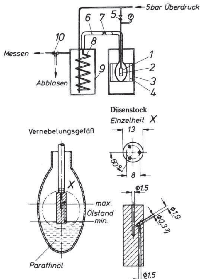
Bild 2. Schematischer Aufbau des Nebelentwicklers für die Erzeugung des Prüfaerosols 1 (Paraffinölnebel)
