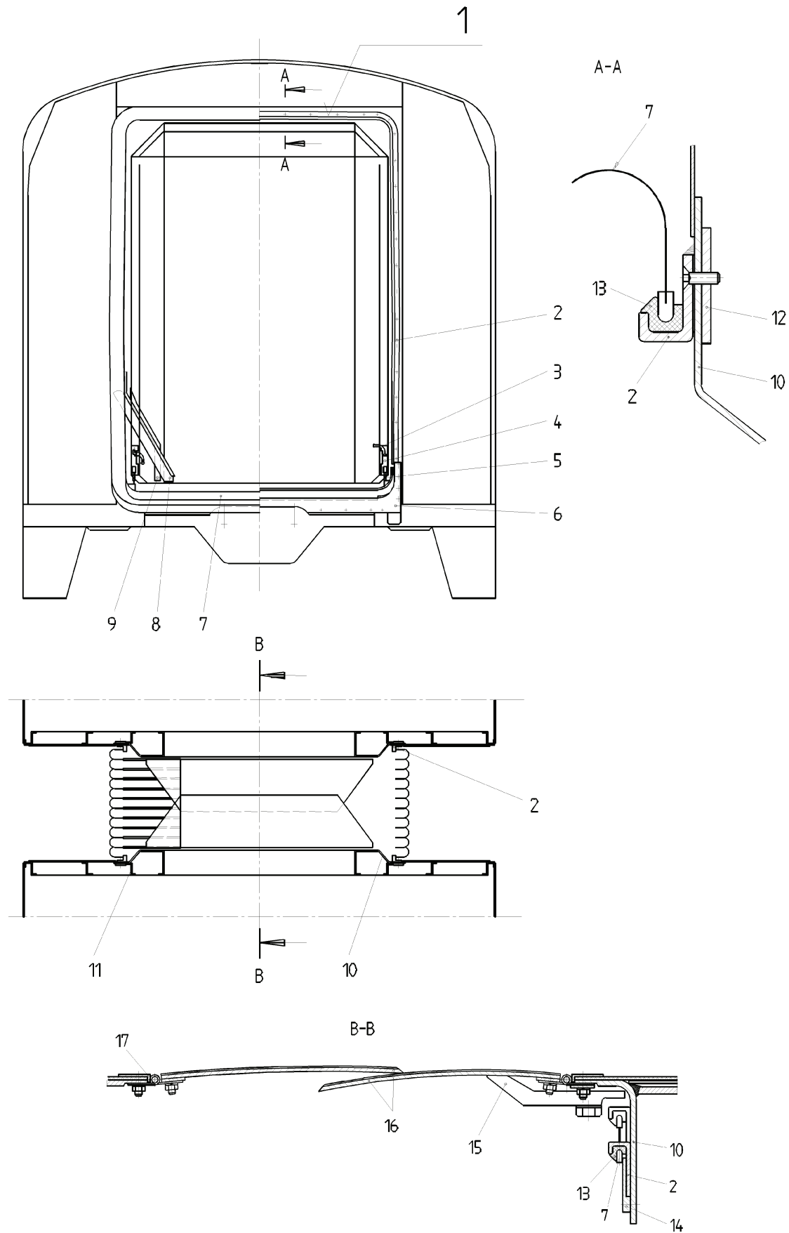
Bild 1 – Übergangseinrichtung
