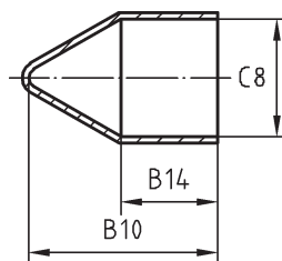
Bild 8 — Schleifkappe, kegelig
