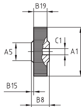
Bild 12 — Lamellenschleifscheibe
