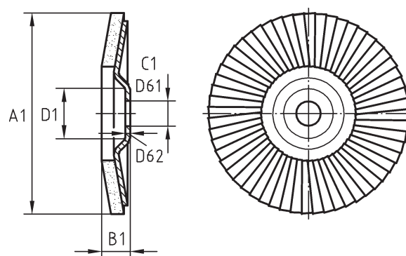
Bild 16 — Fächerschleifscheibe, schräg
