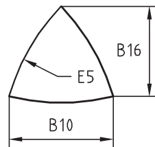
Bild 4 — Schleifblatt, dreieckig
