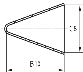
Bild 9 — Schleifkappe, spitz
