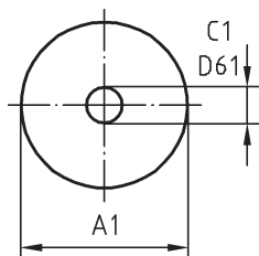
Bild 3 — Schleifblatt, rund
