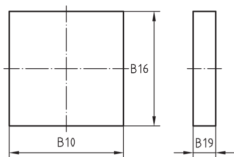
Bild 15 — Schleifklotz
