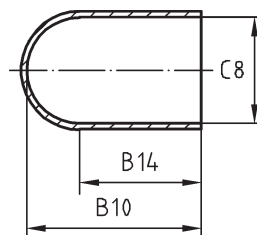
Bild 10 — Schleifkappe, rund
