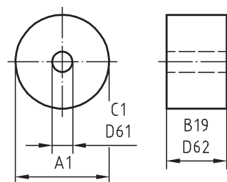
Bild 14 — Vliesschleifscheibe/-walze
