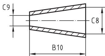
Bild 7 — Schleifhülse, kegelig
