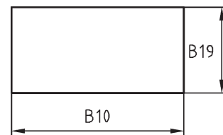
Bild 2 — Schleifblatt, rechteckig
