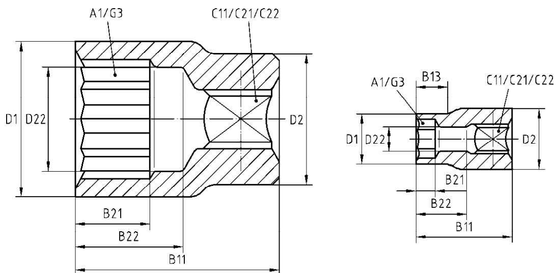
Bild 1 — Steckschlüsseinsätze mit Innenantrieb, für Schrauben mit Außenprofil
