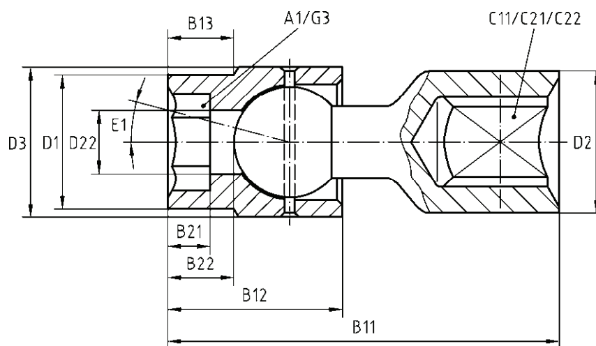
Bild 2 — Steckschlüsseinsätze mit Innenantrieb und mit Gelenk, für Schrauben mit Außenprofil
