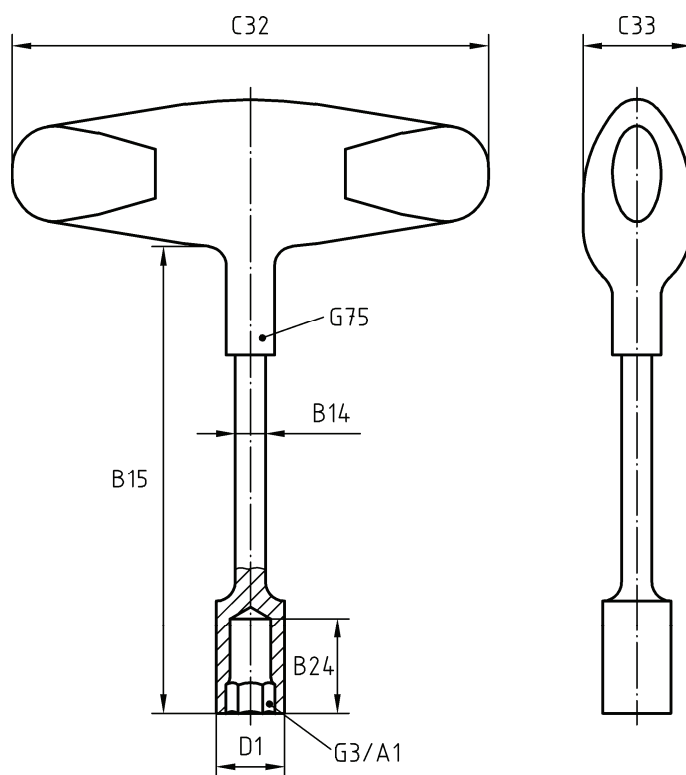
Bild 2 — Schraubendreher und Steckschlüssel mit Quergriff
