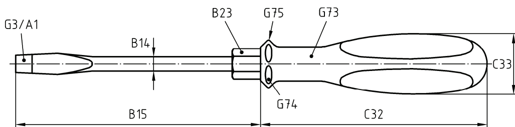
Bild 1 — Schraubendreher und Steckschlüssel
