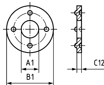
Bild 8 — ID = DIN-AAA768 Scheiben mit Schweißbuckel
