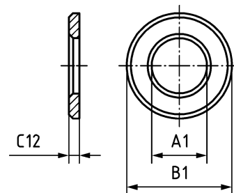
Bild 4 — ID = DIN-AAA765 Scheiben mit Außen- und Innenfase
