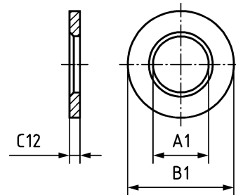
Bild 2 — ID = DIN-AAA763 Scheiben mit Innenfase
