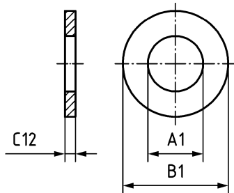
Bild 1 — ID = DIN-AAA762 Scheiben, flach
