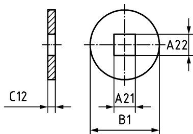
Bild 5 — ID = DIN-AAA766 Scheiben mit Innenvierkant/Rechteck
