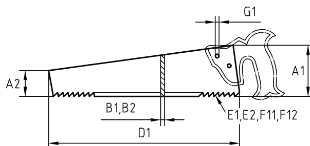
Bild 1 — Fuchsschwanzsägeblatt
