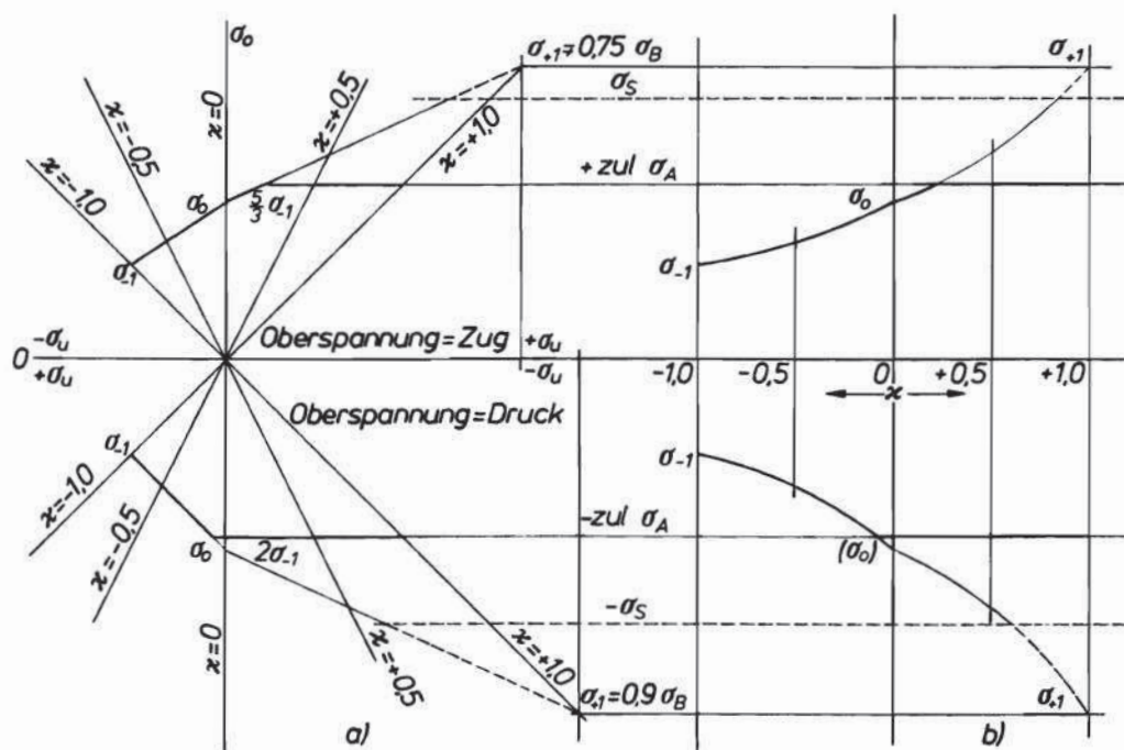
Bild 3. Zusammenhänge zwischen zul \sigma_{Be,x} und zul \sigma_{Be,x=-1}
