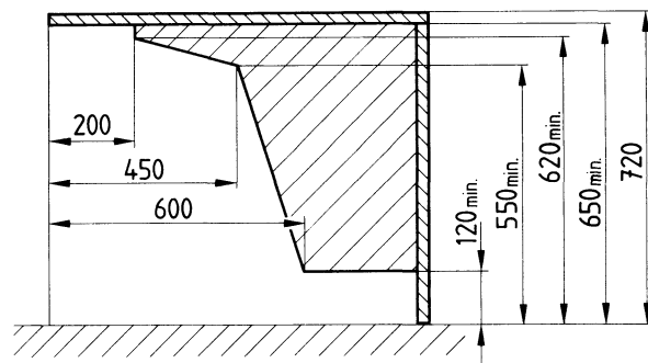
Bild 1. Mindestmaße des Beinraumes von Schreibtischen und Bildschirmarbeitstischen
