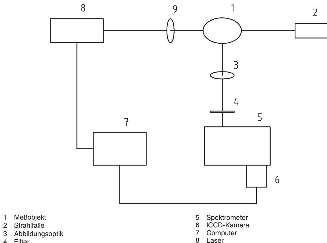
Bild 1: Schematische Darstellung für die Temperaturbestimmung mit Raman-Streuung
