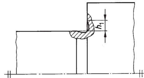
Bild 3: Welle mit Freistich
