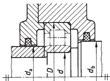
Bild 4: NU
