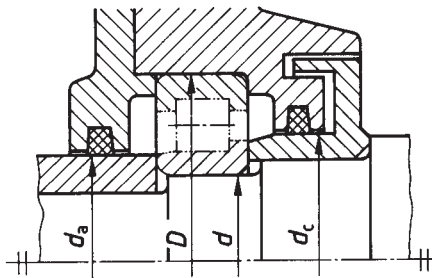
Bild 5: NJ
