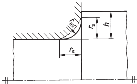
Bild 2: Welle
