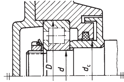
Bild 6: NUP
