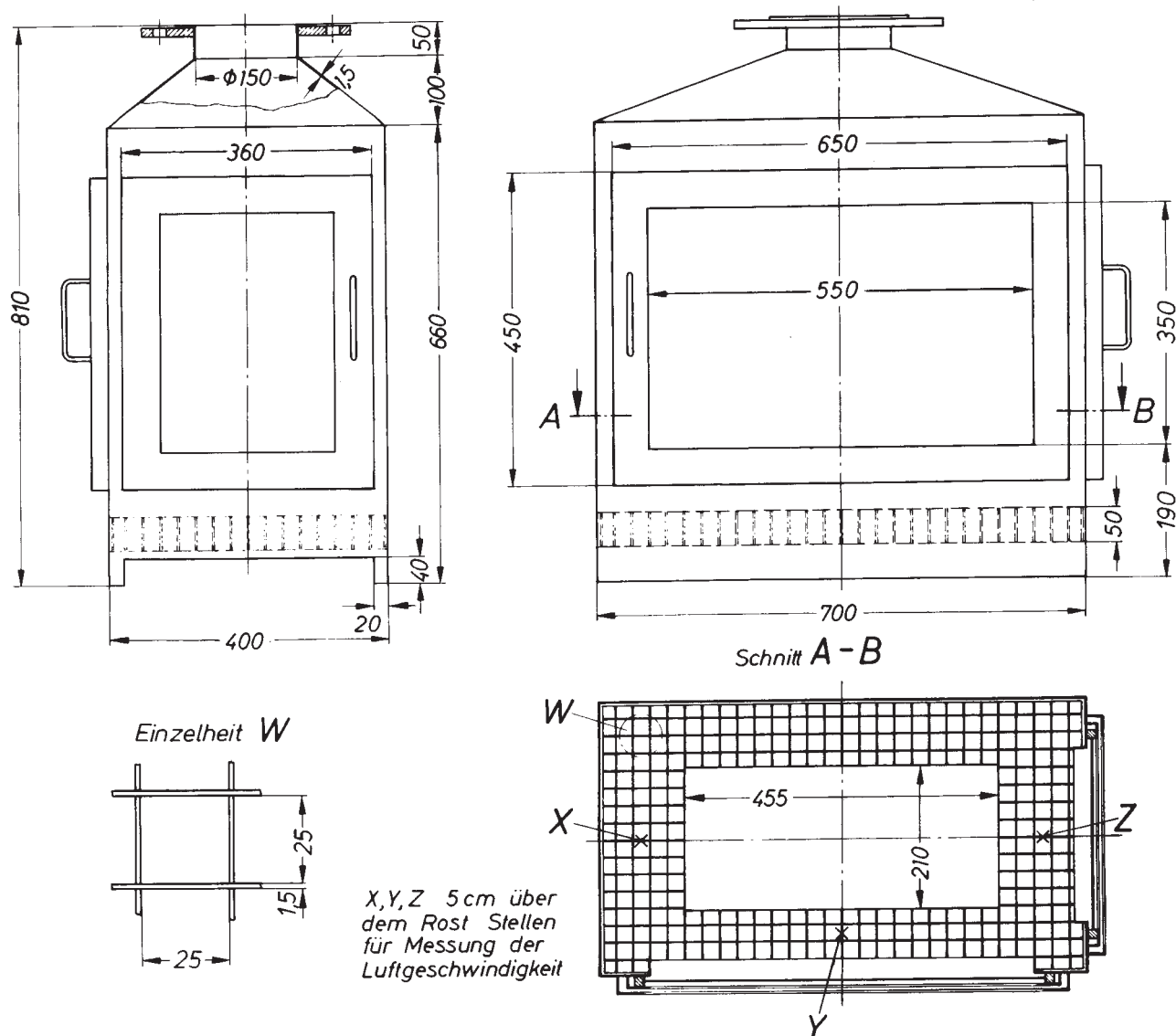
Bild 1. Brennkasten
