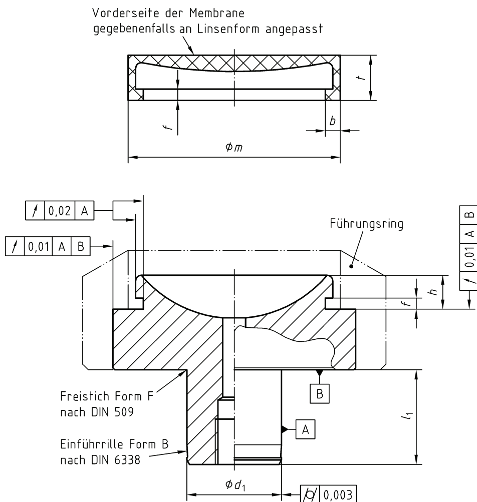
Bild 1 – Werkstückaufnahme mit Membranen (M)
