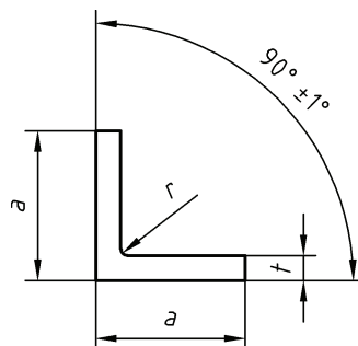
Bild 1 — Blanker gleichschenkliger scharfkantiger Winkelstahl
