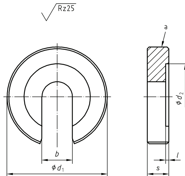
Bild 1 — Vorsteckscheibe
