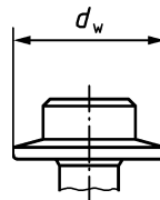
Bild 2 — Senkkopf
