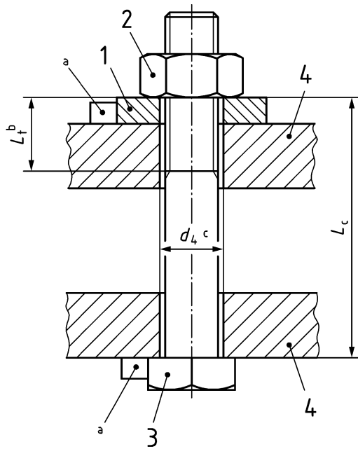
Prüfung der Mutter
