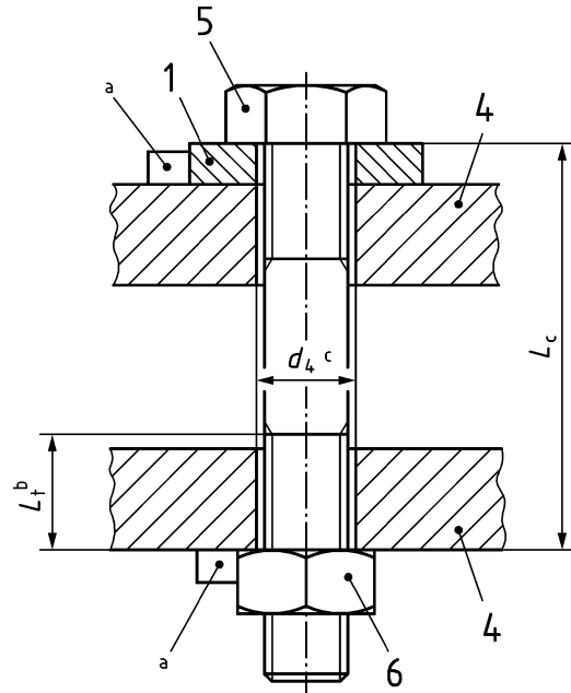
Prüfung der Schraube
