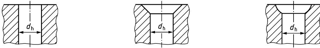
Bild 1 — Durchmesser des Durchgangslochs der Scheibe oder der Auflageplatte
