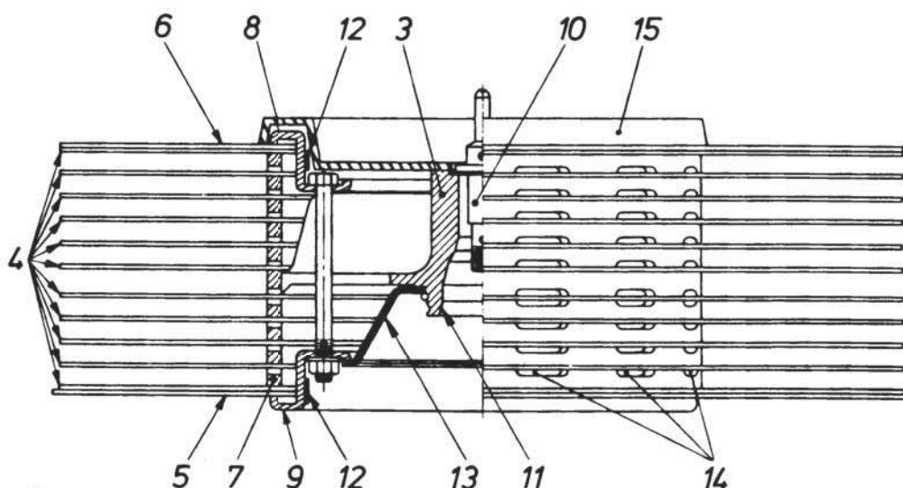
Bild 1. Plattenpaket (Ziffern siehe bei Bild 2)
