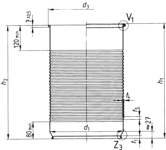
Deckelbehälter mit Mantelausführung M10
