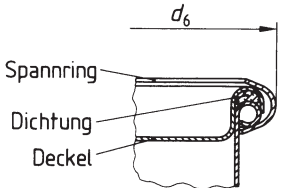
Einzelheit V1
