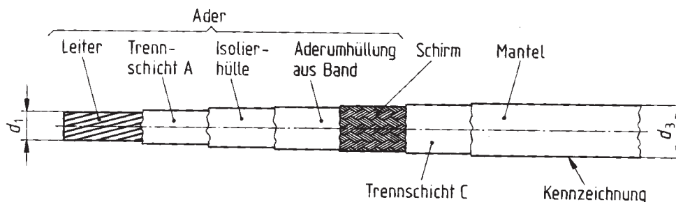
Bild 1: Einadriges Kabel
