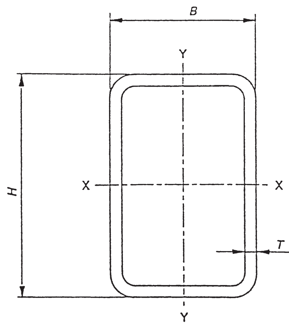
Bild 10: Hohlprofil mit rechteckigem Querschnitt (siehe Tabelle 7)
