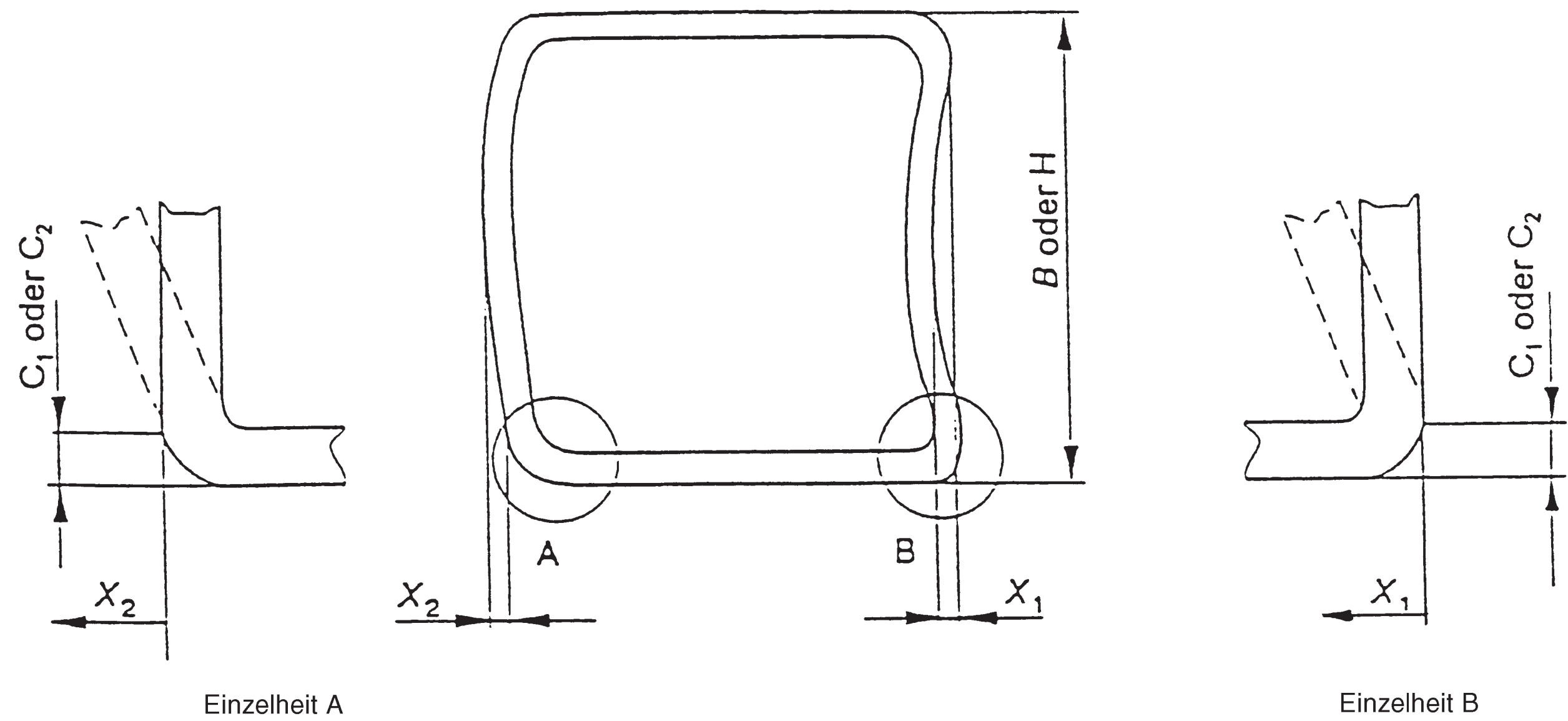
Bild 2: Messung der Konkavität bzw. Konvexität von Hohlprofilen mit quadratischem oder rechteckigem Querschnitt
