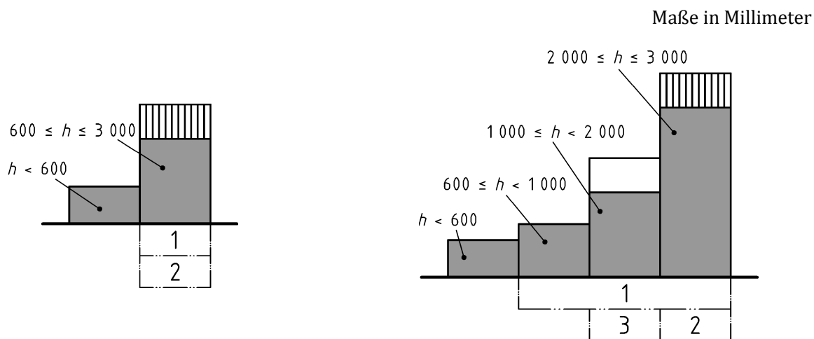
a) Absturzsicherung für leicht zugängliche Geräte
