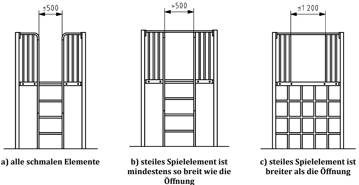
Bild 10 — Zugangs- und Ausgangsöffnungen in Brüstungen für steile Spielelemente
