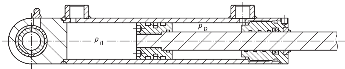
Bild 8 — Zugzylinder oder Druckzylinder mit druckbeaufschlagter kolbenstangenseitiger Kammer
