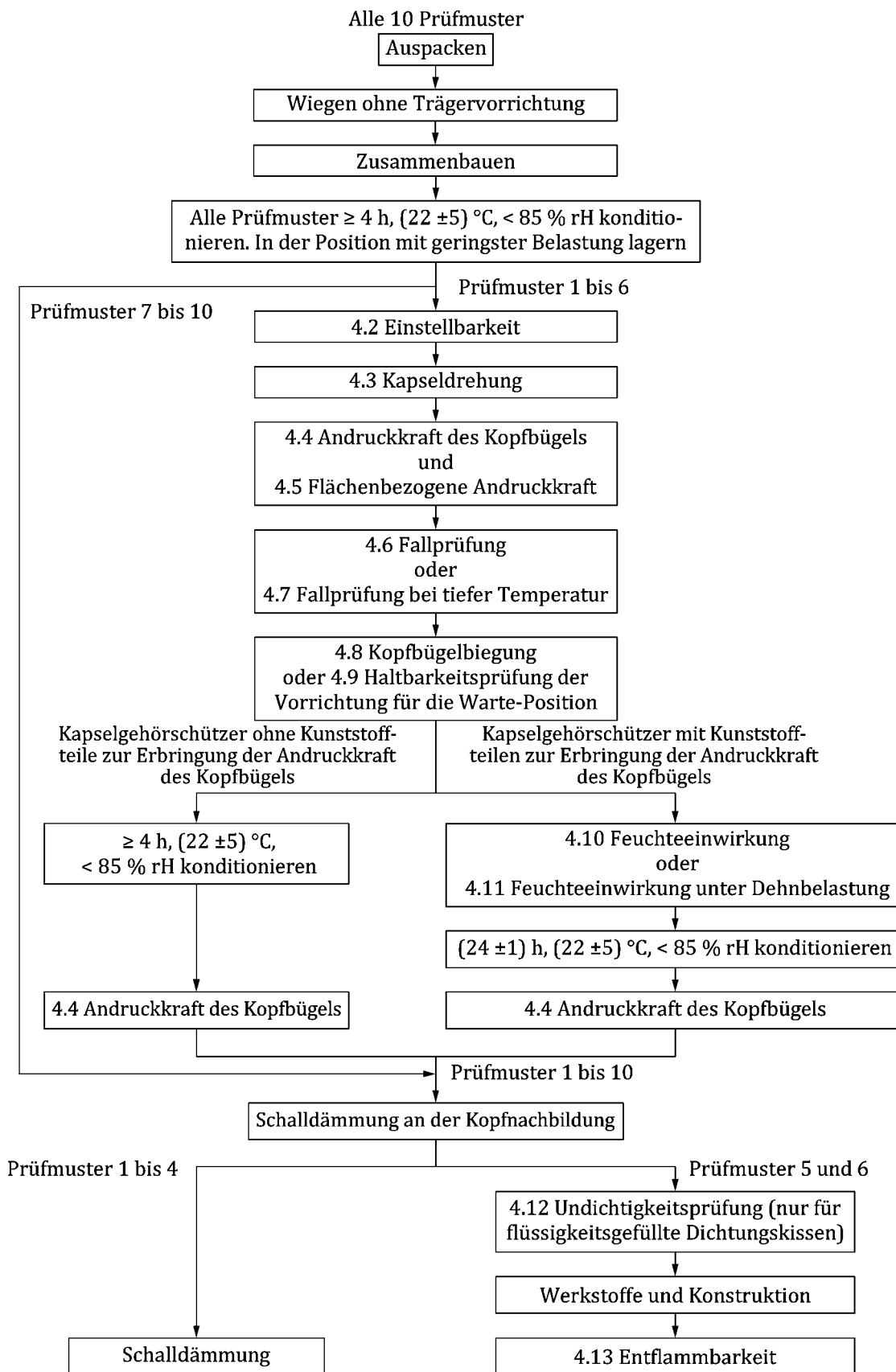
Bild 2 — Flussdiagramm des Prüfschemas für befestigte Kapselgehörschützer – Basiskombination
