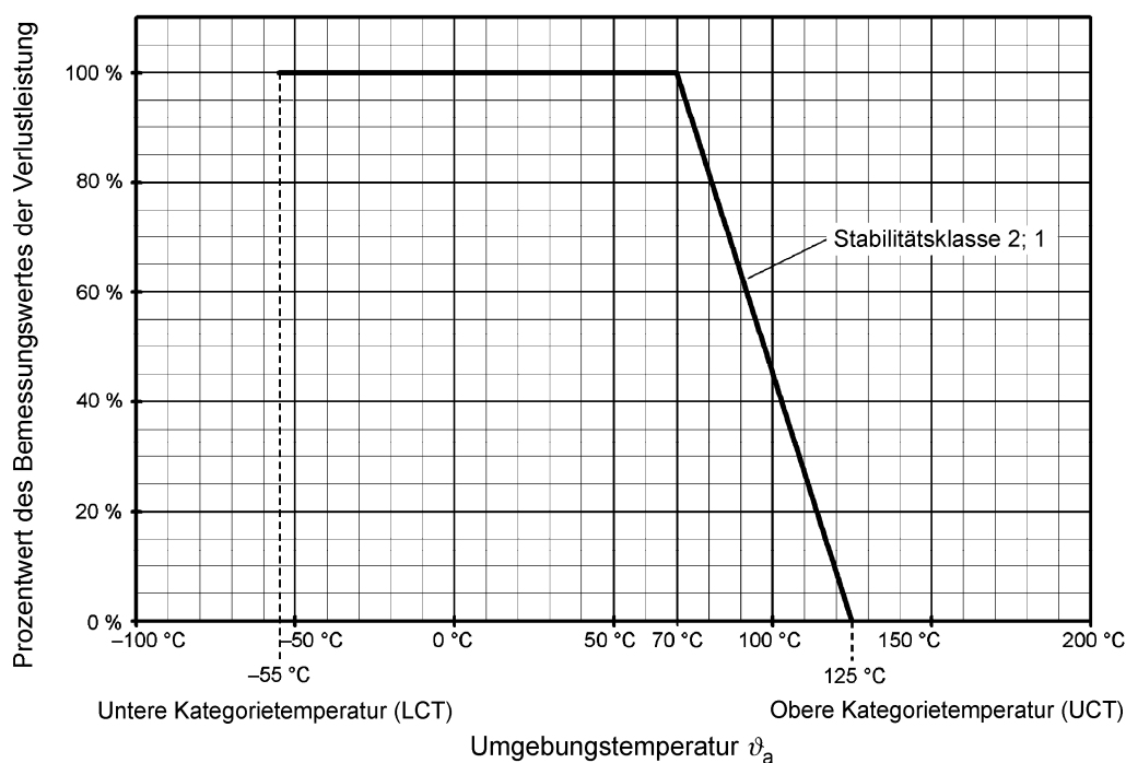
Bild 2 – Lastminderungskurve
