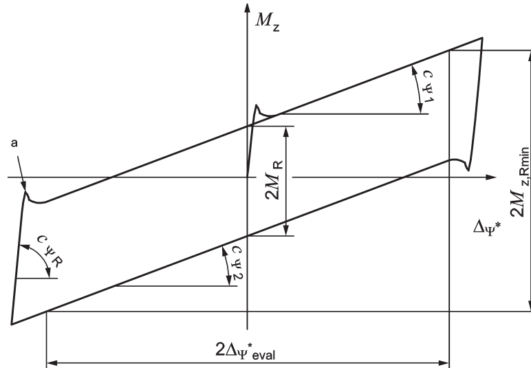
Bild 6 — Drehgestell-Ausdrehdiagramm
