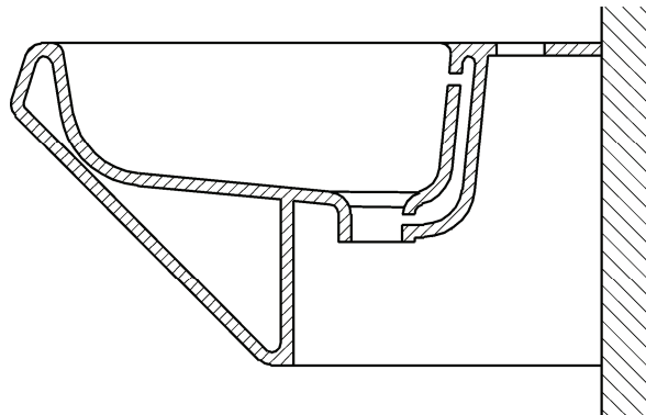
Bild 1 — Wandhängendes Sitzwaschbecken
