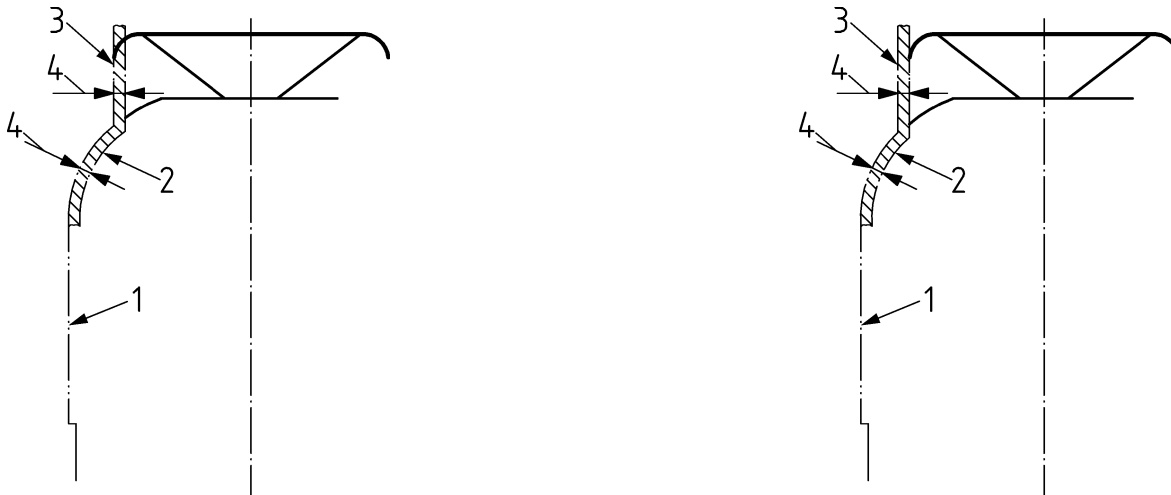
a) Stromabnehmer mit isolierten Auflaufhörnern
